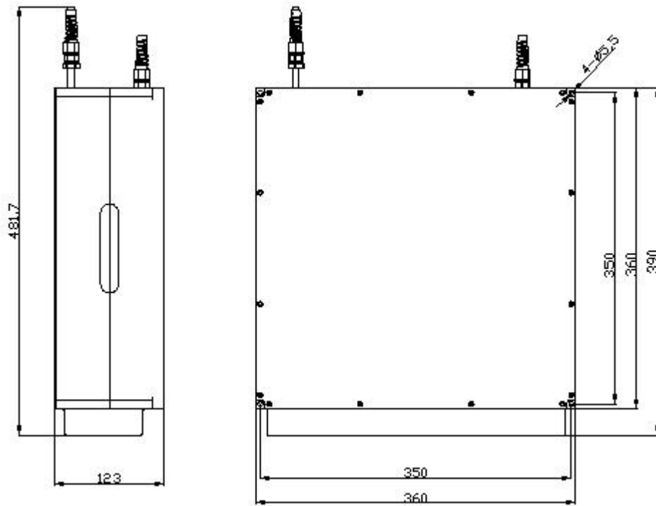
图 1 激光器尺寸图（单位 mm）
