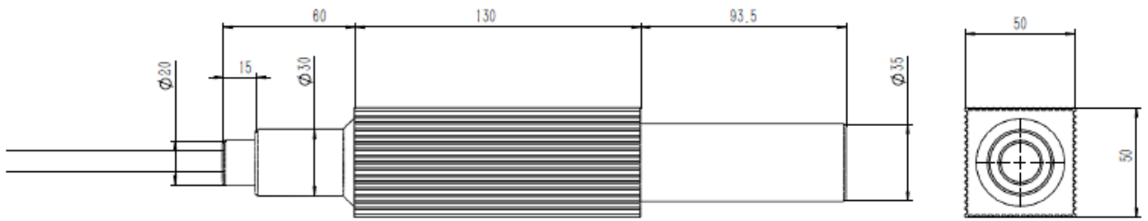
图 2 输出光隔离器尺寸图（单位 mm）
