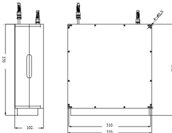
图 1 激光器尺寸图 (单位 mm)
