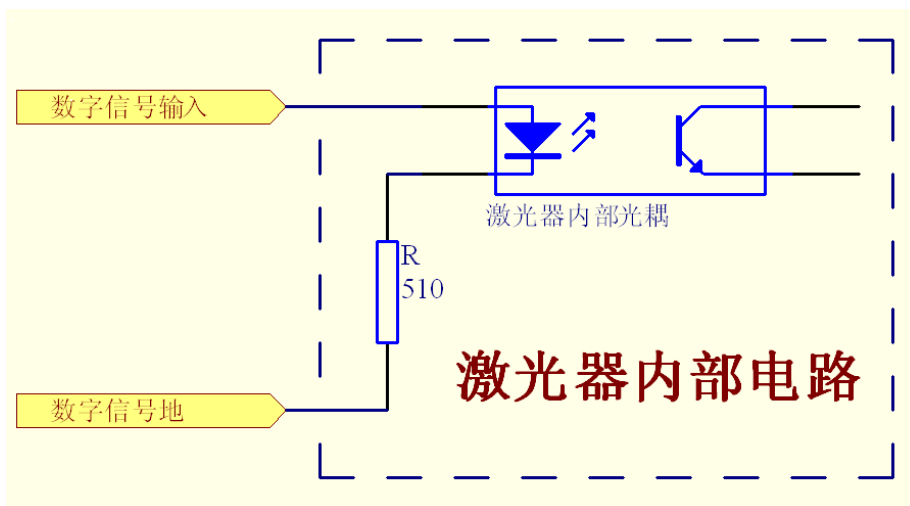
图 6 输入控制信号内部结构图
