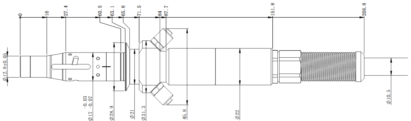
图 7 IQB 输出光缆 (单位: mm)
