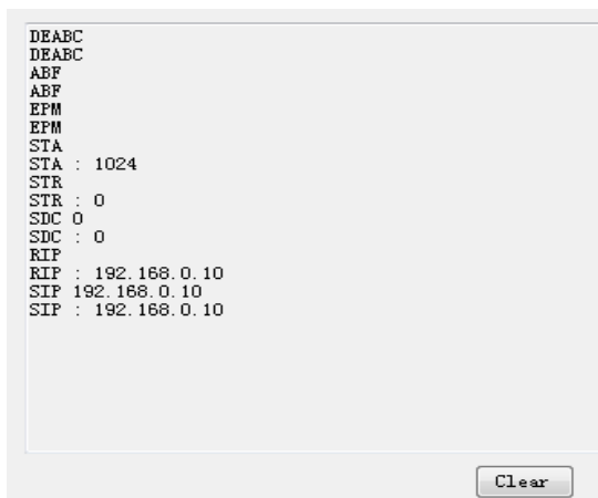
图 A.26 主界面——通讯命令显示 每点击一次按钮后该显示区显示当前按钮对应的命令，同时显示激光器的回应信息，便于客户自己开发控制系统。
