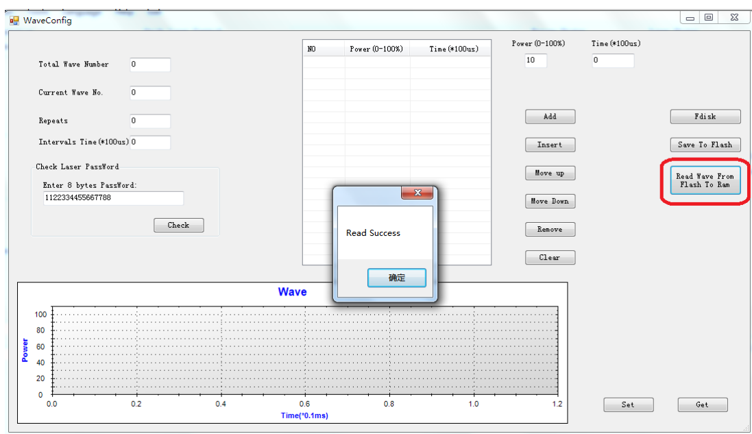
图 A.30 读取波形文件到单片机 RAM
