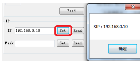
图 A.14 主界面——激光器 IP 设置
