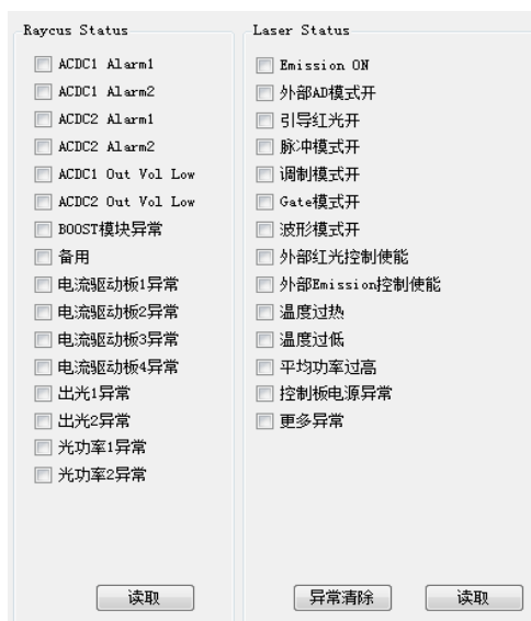
图 A.25 主界面——激光器状态显示
