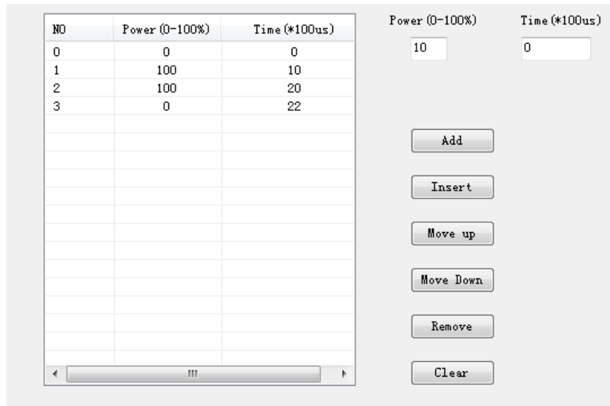
图 A.34 编辑新的波形——描点
