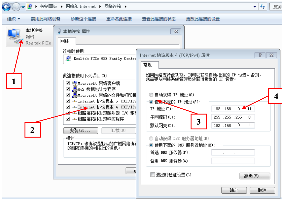
图 A.42 以太网本地连接配置
