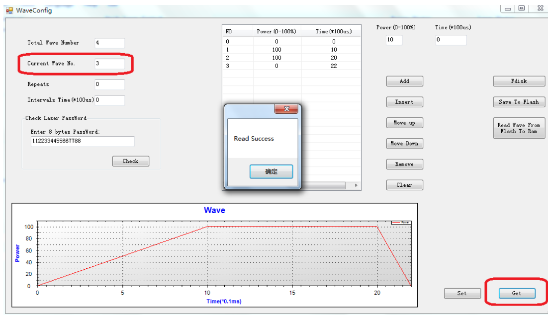
图 A.32 读取波形
