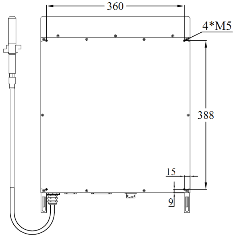
图 6 激光器底部视图(固定孔位)
