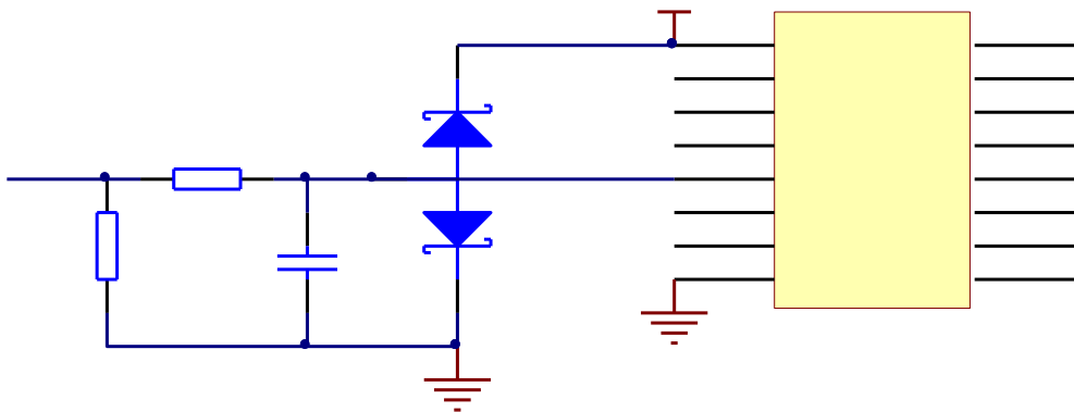
图 11 数字信号输入接口电路
