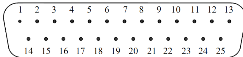
图 15 DB25 控制接口示意图
