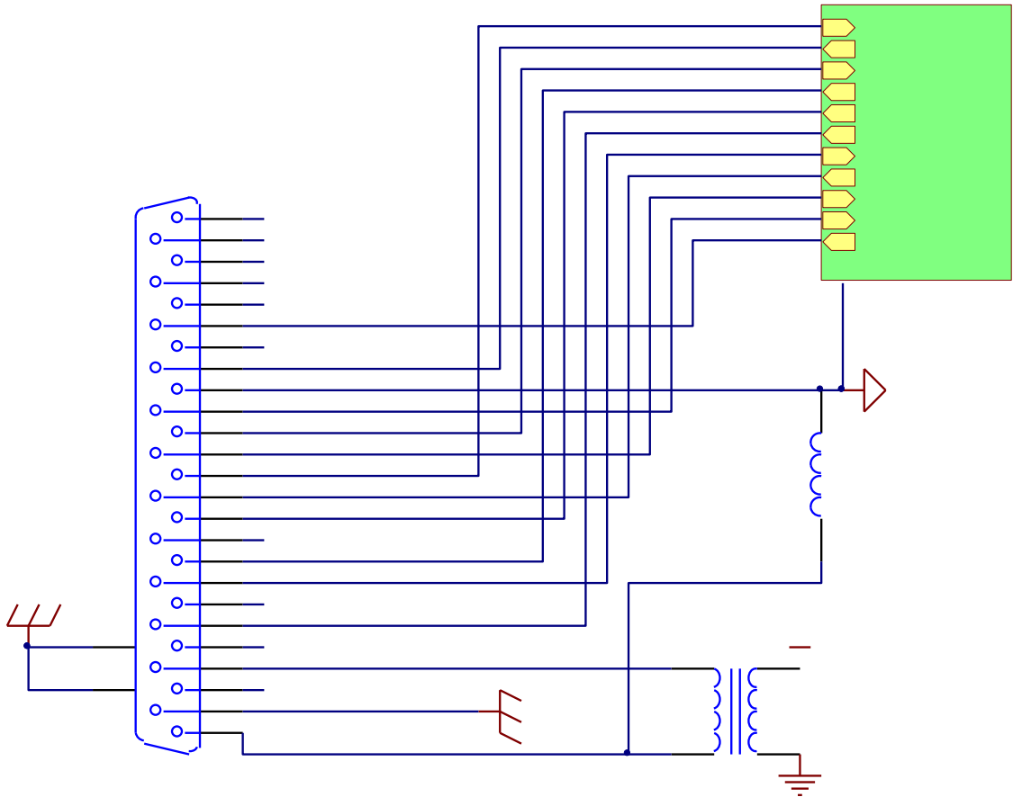
图 10 DB25 控制接口信号流向
