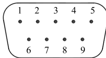
图 16 RS-232 串口示意图
