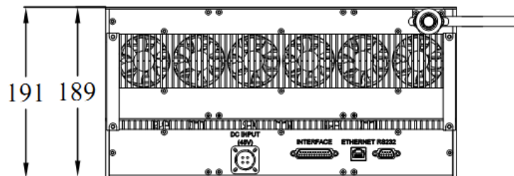
图 2 激光器前视图
