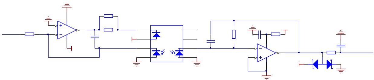
图 14 模拟量信号输出接口电路
