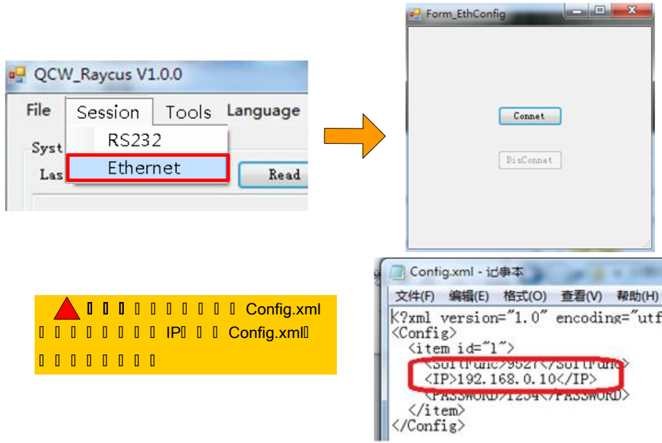
图 A.6 以太网通讯
