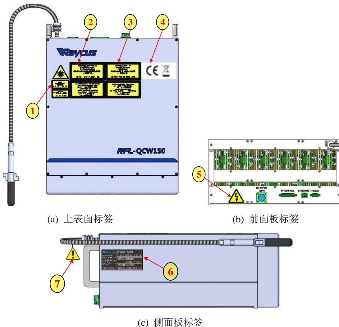
图 1 安全标识位置
