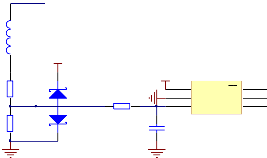
图 13 0-4V 模拟信号输入接口电路
