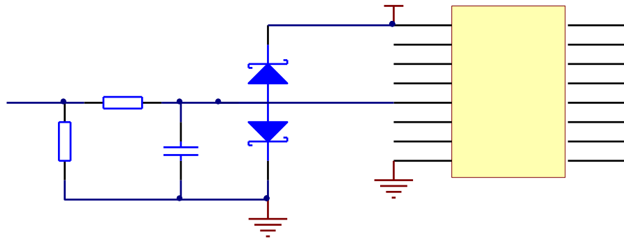
图 12 数字信号输出接口电路
