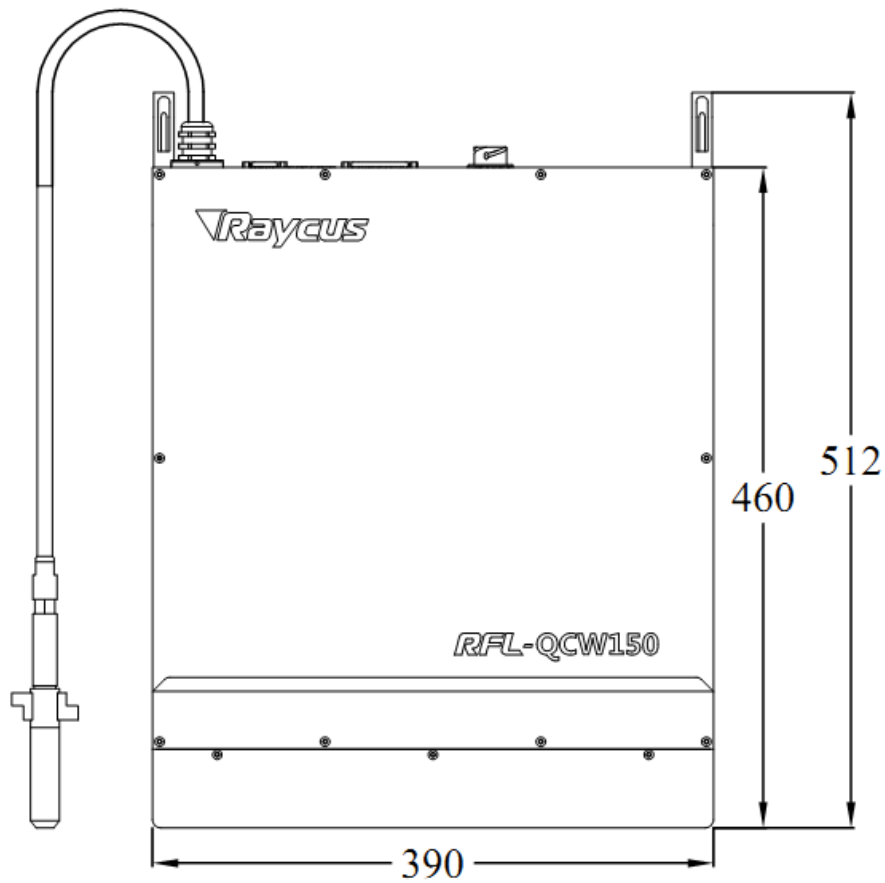
图 5 激光器俯视图
