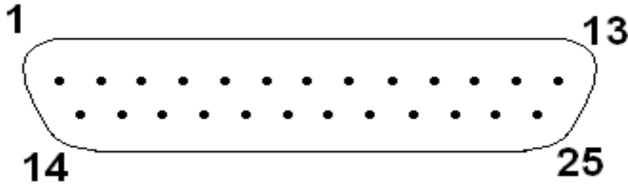
图 5 控制接口图
