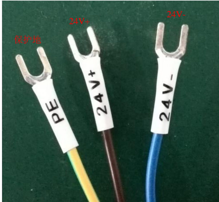
图 3 电源线接头定义
