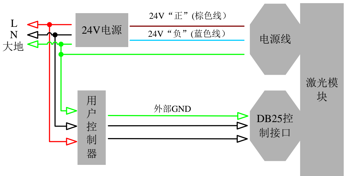
图 4 电气连接图
