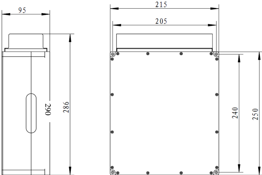
图 1 激光器尺寸图（单位 mm）
