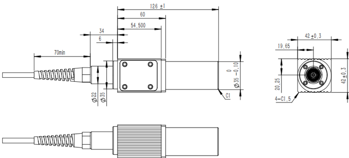
图 2 输出光隔离器尺寸图（单位 mm）
